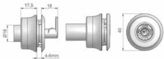
Technische tekening
