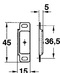
OMSCHRIJVING ZEER DUNNE MAGNEET MET ZELFKLEVENDE TEGENPLAAT
