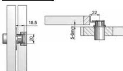
Technische tekening
