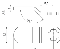
Sluithaak gebogen klein
