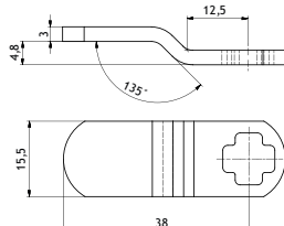
Sluithaak gebogen klein
