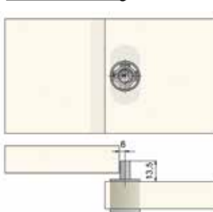
Technische tekening
