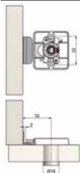
Technische tekening
