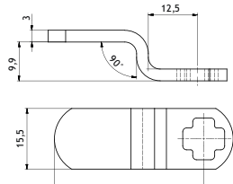
Sluithaak gebogen groot
