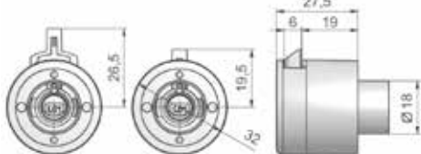
Technische tekening
