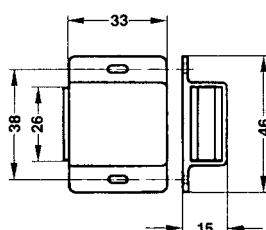
OMSCHRIJVING (•) BEWEEGLIJKE TEGENPLAAT VOOR ARTIKELS 2506-0704, 2506-0700
