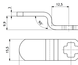
Sluithaak gebogen groot
