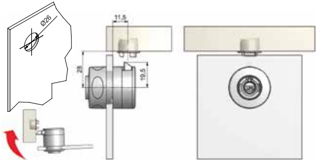
Technische tekening
