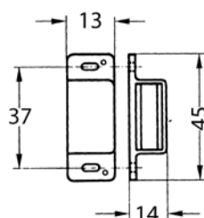
OMSCHRIJVING MAGNEET ZONDER TEGENPLAAT (•)
