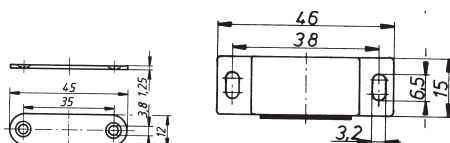
OMSCHRIJVING MAGNEET MET METAALPLAAT.
