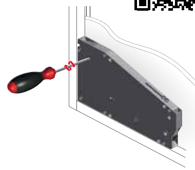
BUITENKANT VAN DE KAST
