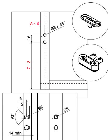
Boorschema aluminium deuren
