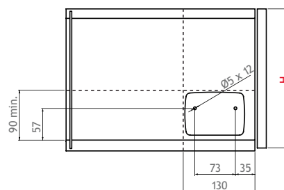
Boorschema zijpanelen
