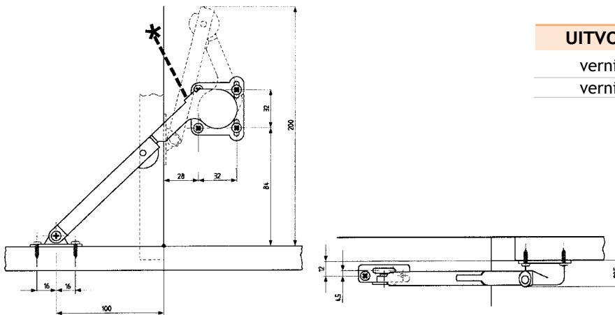
Cea-lift 601 valschaar
