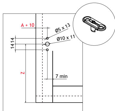
Boorschema houten deuren
